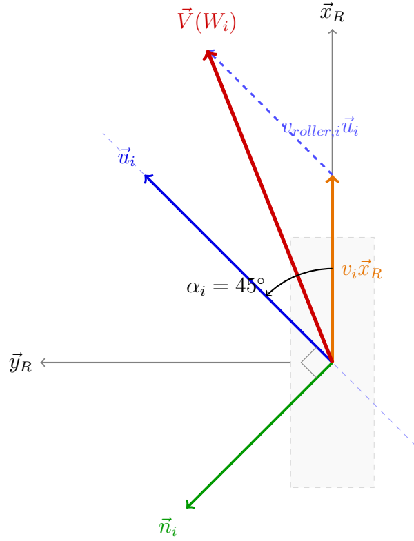
FIGURE 9 – Modélisation géométrique des vitesses et projection de contrainte.
