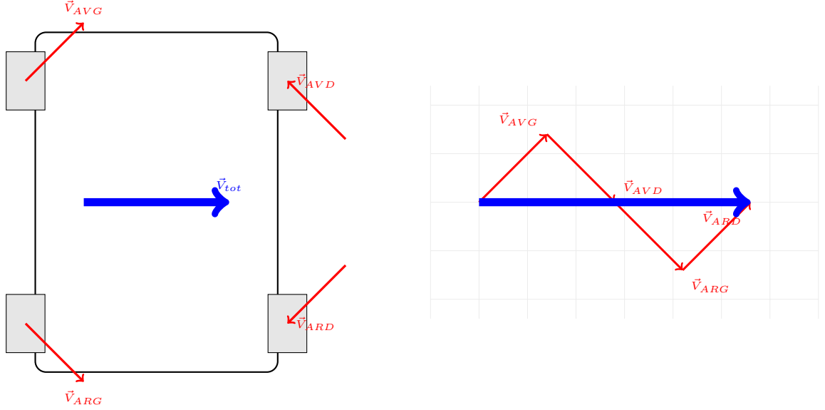
FIGURE 11 – Comportement latéral (Axe Y). L'opposition des forces avant/arrière s'annule, ne laissant subsister que le déplacement latéral résultant.
