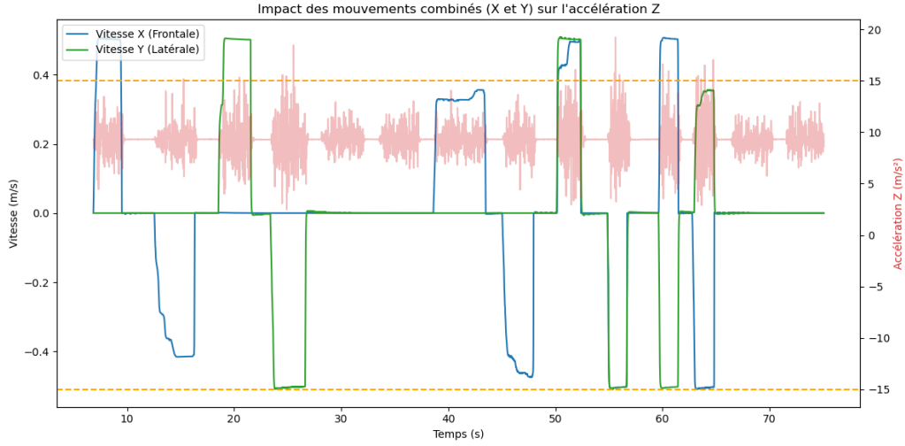
FIGURE 6 – Superposition temporelle des cinématiques de translation et des réponses vibratoires du châssis.
