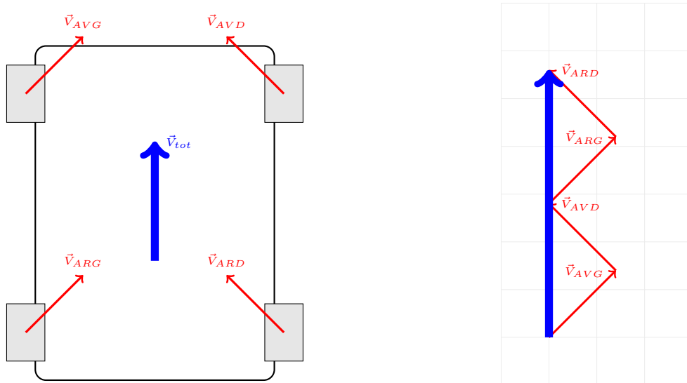
FIGURE 10 – Comportement longitudinal (Axe X). Les efforts se cumulent vers l'avant tandis que les poussées latérales s'annulent géométriquement.
