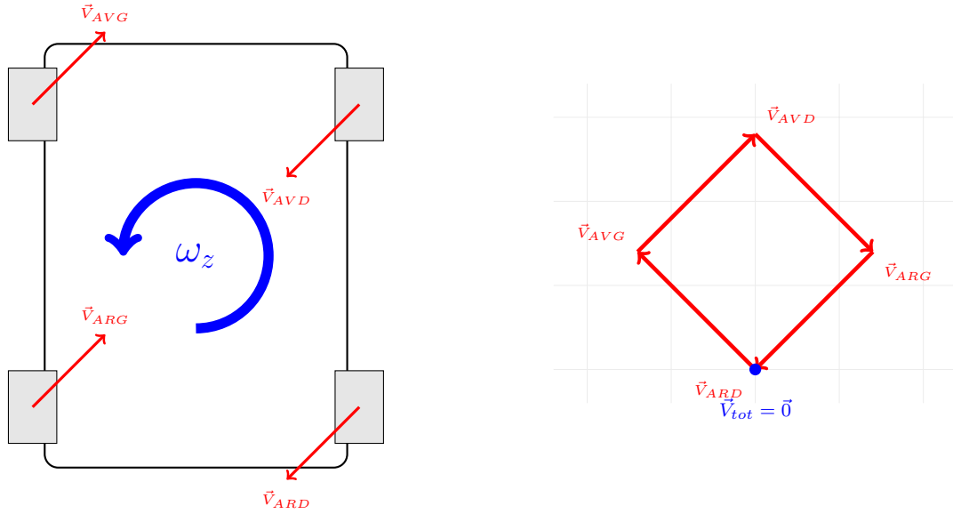
FIGURE 12 – Comportement en rotation pure ( \omega_z ). Le bouclage fermé démontre analytiquement l'absence de toute translation résiduelle du châssis.
