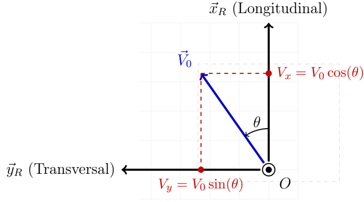
FIGURE 14 – Représentation vectorielle du cap oblique \theta . La vitesse cible V_0 se projette sur l'axe frontal ( V_x ) et sur l'axe latéral ( V_y ) selon l'orientation angulaire du vecteur de translation demandé par l'utilisateur.
