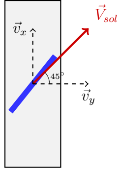
FIGURE 7 – Décomposition de la vitesse au sol. Le rectangle gris représente la roue, le trait bleu le galet orienté à 45^\circ .
