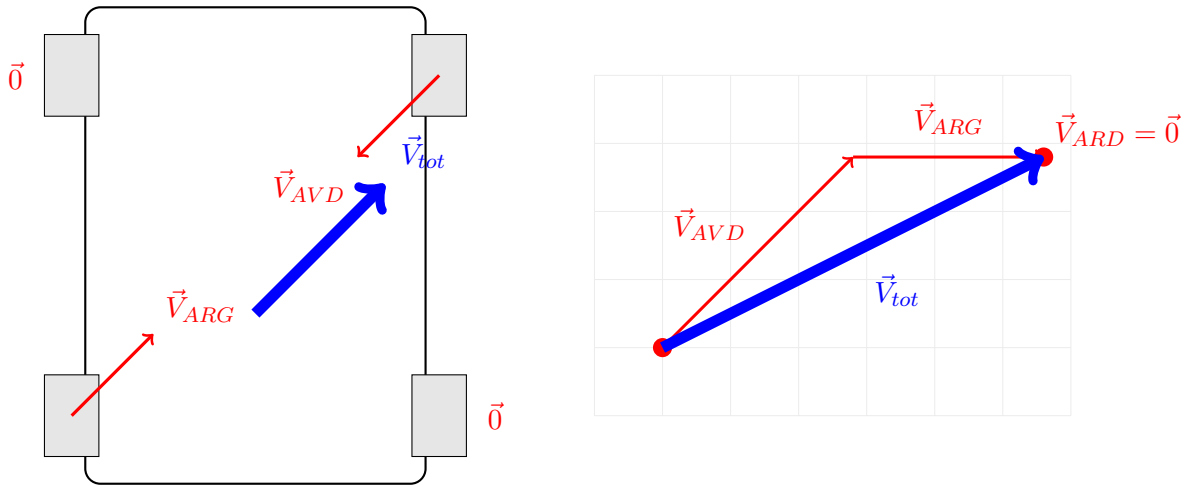
FIGURE 13 – Comportement oblique singulier ( \theta = 45^\circ ). L'arrêt complet de deux roues reporte toute la charge sur la seconde diagonale, provoquant d'importants sauts de charge mécanique.
